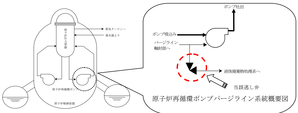
原子炉再循環系 系統概要図
