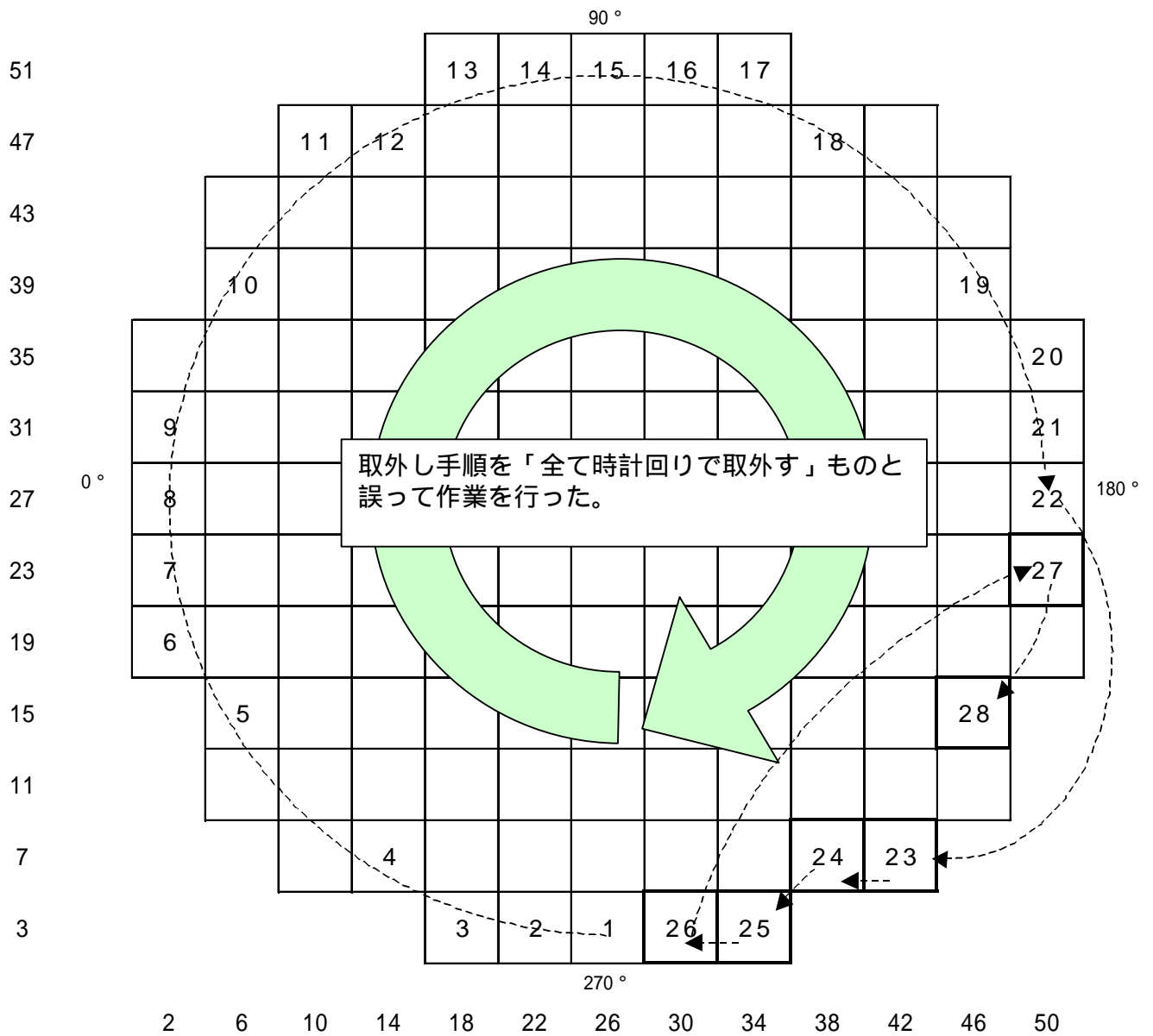
女川2号機 第6回定期検査時(シュラウド点検)の制御棒取外し手順(追加分) 取付けは、取り外しと逆の順番(不規則パターン)
