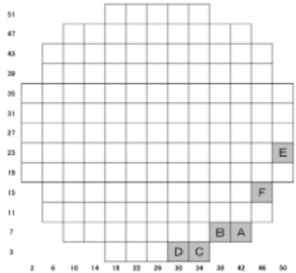
入れ違っていた制御棒の配置
