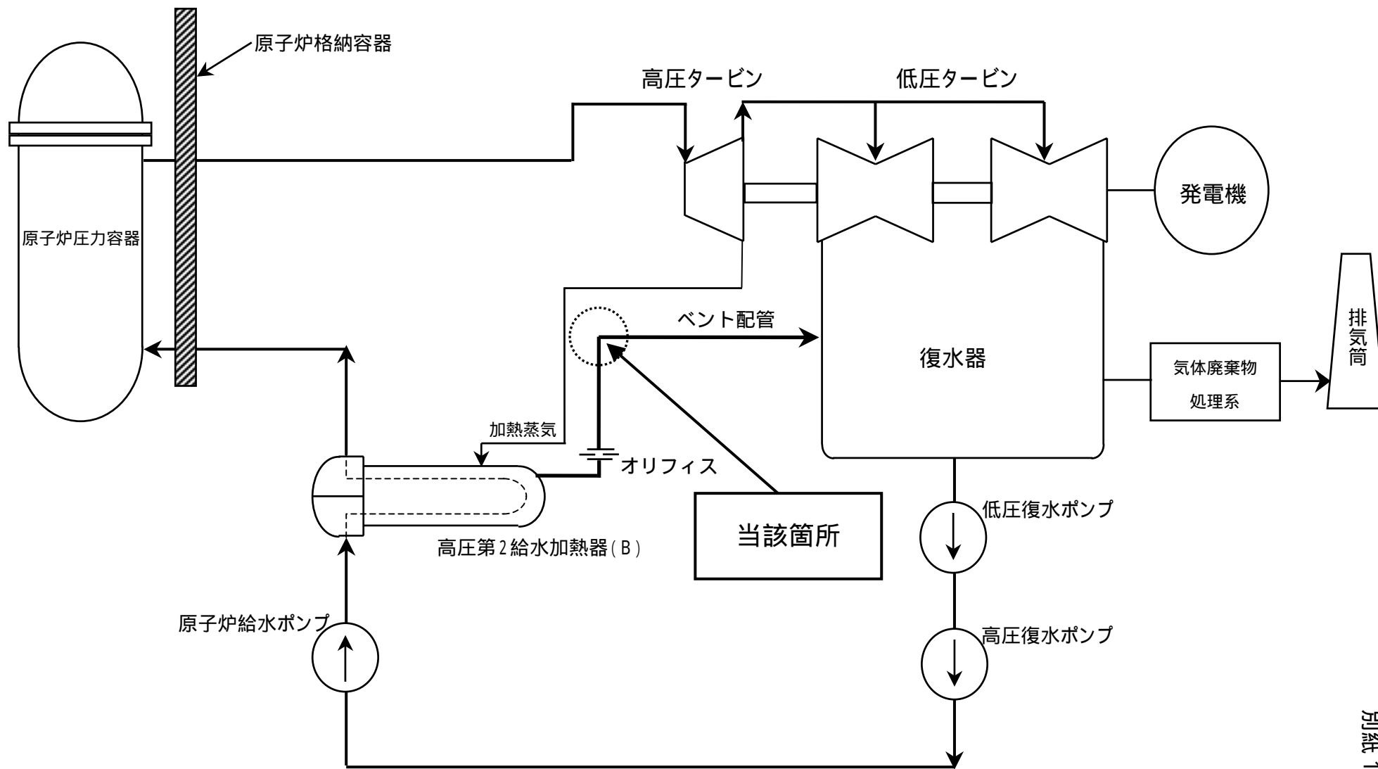
高圧第2給水加熱器(B)ベント配管 概念図
