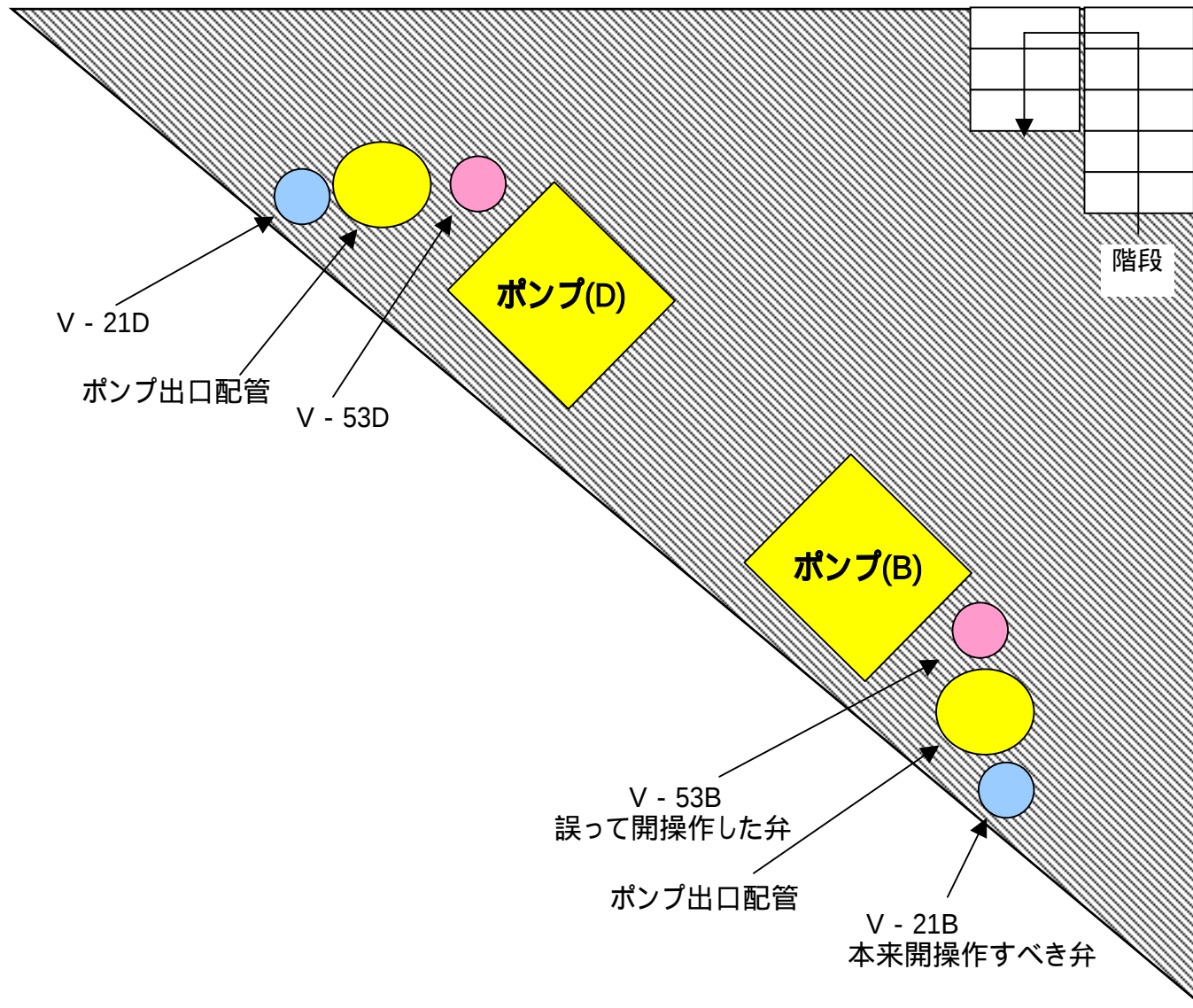
図-3 RHRポンプ(B・D)室(地下中2階)弁配置
