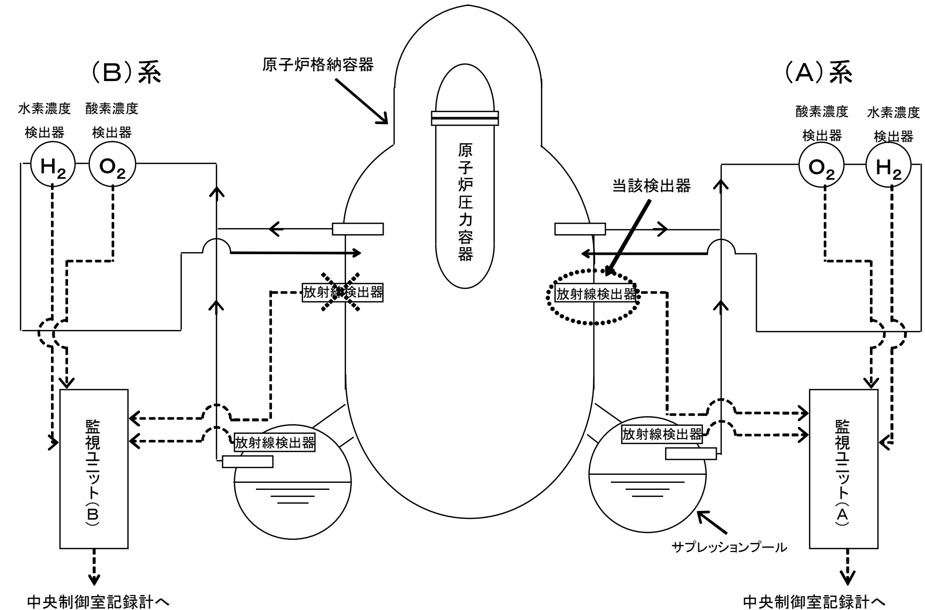
格納容器内雰囲気モニタ系 系統図
