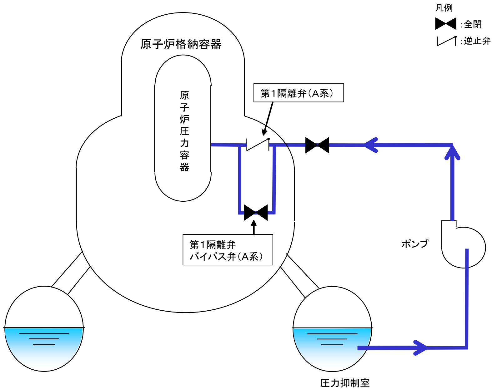
低圧注水系 系統概要図
