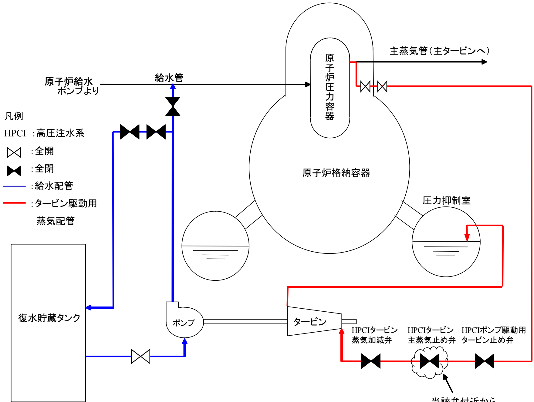
高圧注水系 系統概要図
