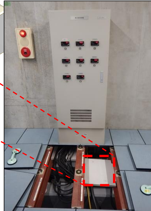
東通原子力発電所1号機 ケーブルの不適切な敷設状態(概要図)
