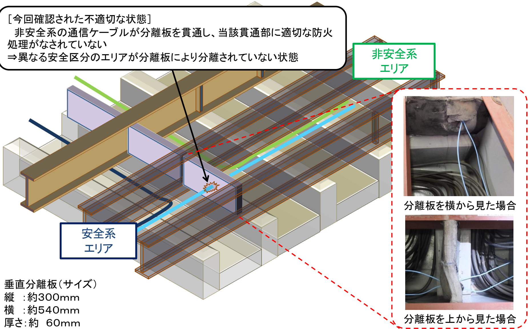
女川原子力発電所3号機 ケーブルの不適切な敷設状態(概要図)
