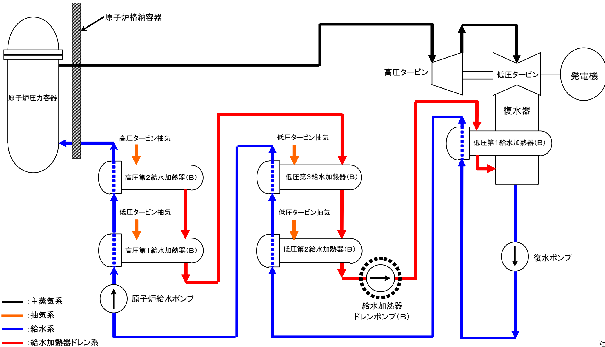
給水加熱器ドレン系 系統概要図
