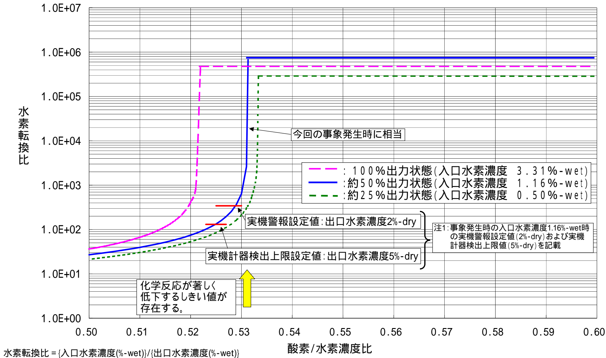
女川3号機の金属触媒における酸素/水素濃度比と水素転換比の関係
