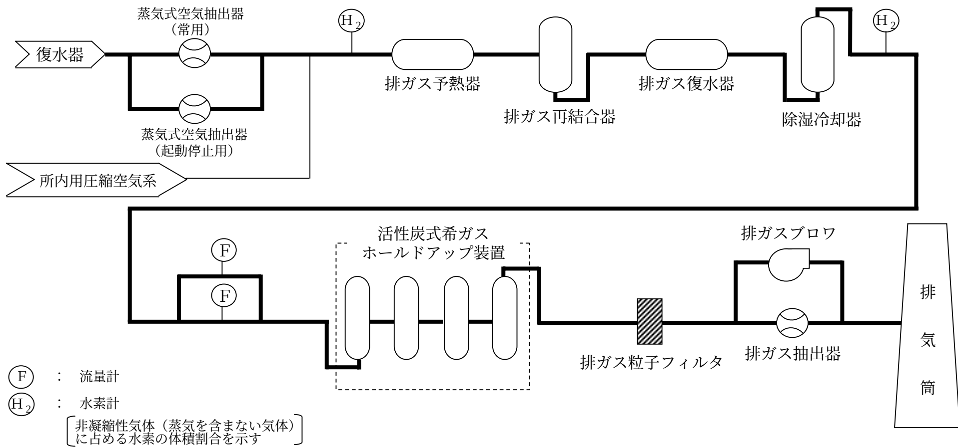
女川原子力発電所 3 号機 気体廃棄物処理系 系統概要図
