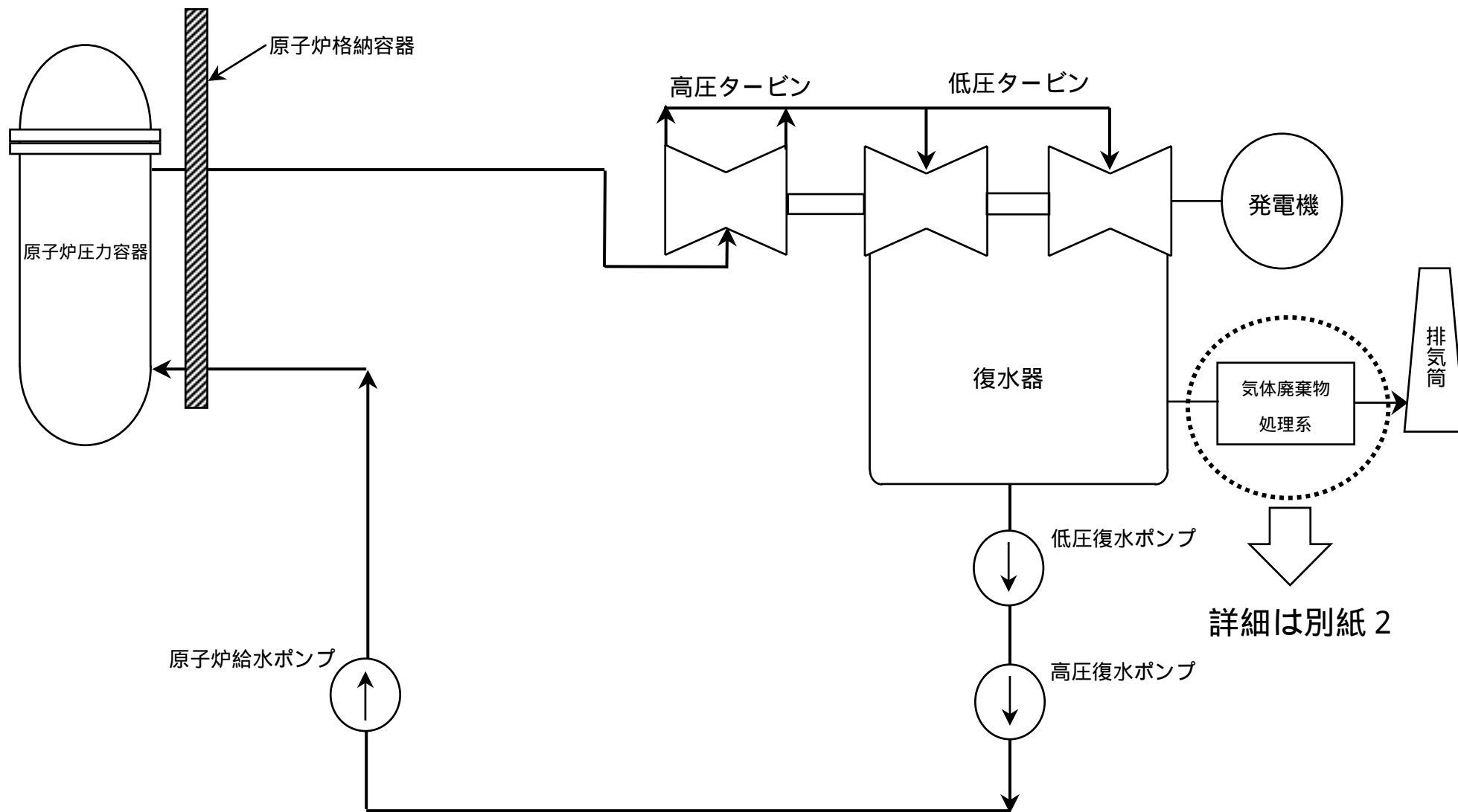
女川原子力発電所 3号機系統図
