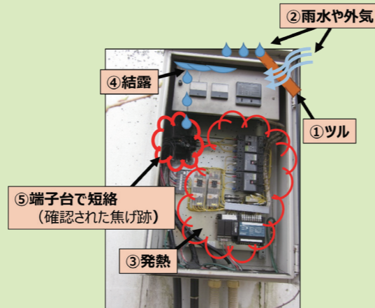
当該分電盤と事象発生イメージ
