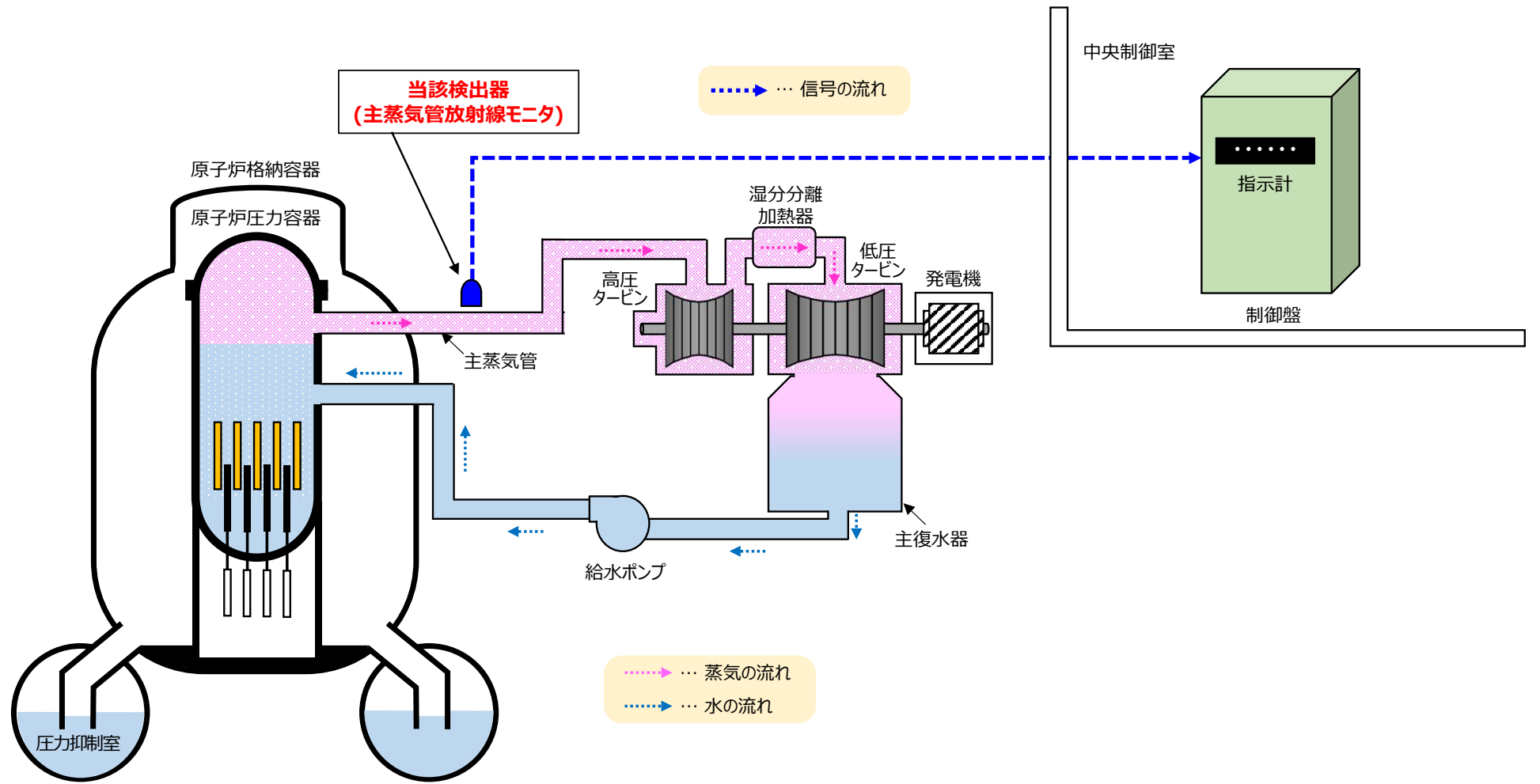
主蒸気管放射線モニタ 概要図
