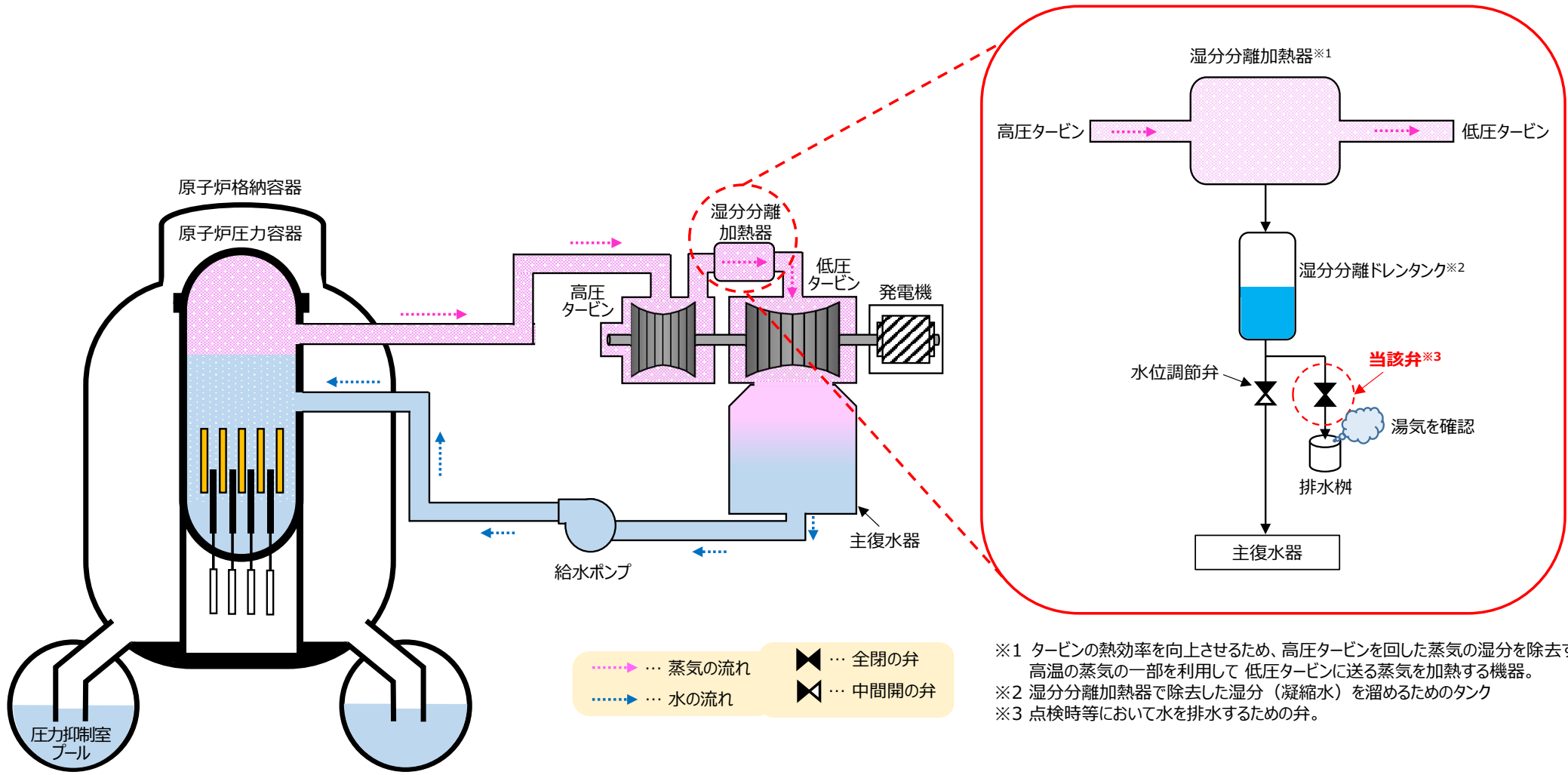
女川原子力発電所2号機 湿分分離ドレンタンク下流の排水柵からの湯気の発生について
