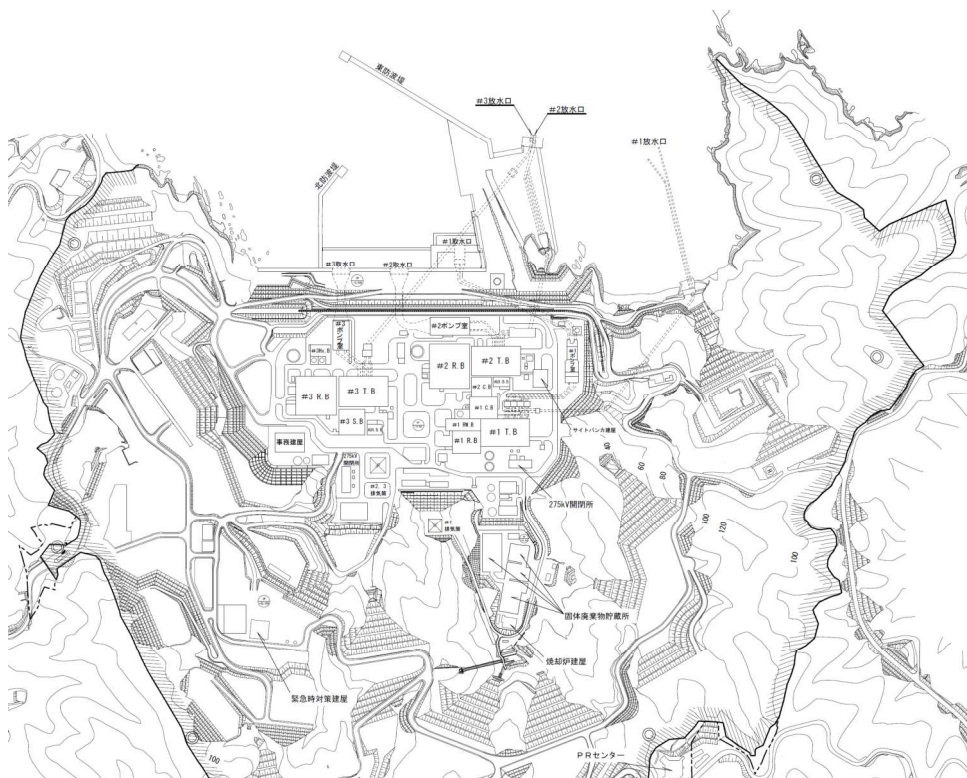
図4-1 女川原子力発電所の配置図
