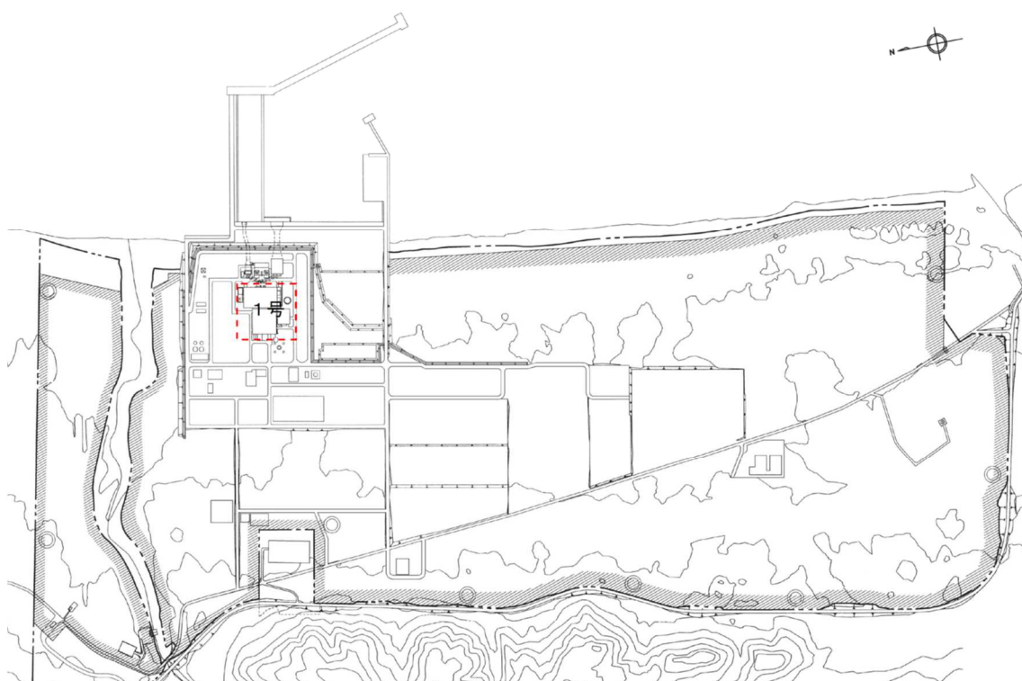
図4-1 東通原子力発電所の配置図
