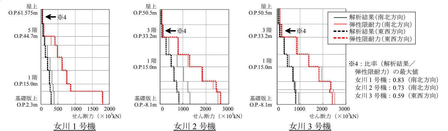
図-5 原子炉建屋の各階毎の耐震壁に作用したせん断力の確認
