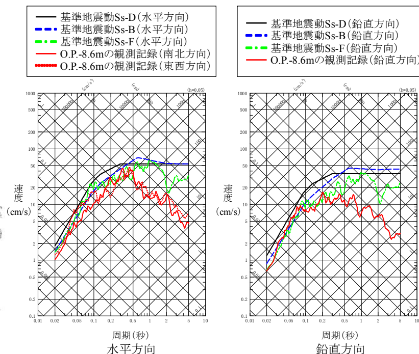
図-3 観測記録の応答スペクトル(岩盤中:解放基盤相当位置)
