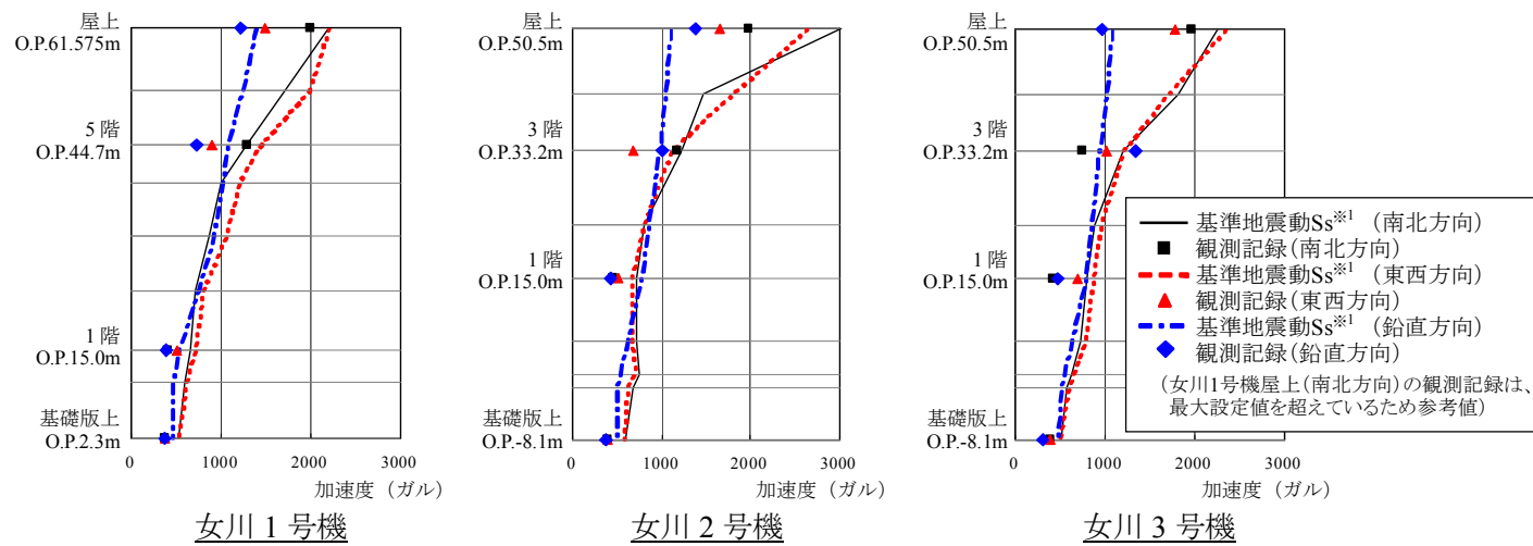
図-1 原子炉建屋の最大加速度分布(建屋観測用地震計)
