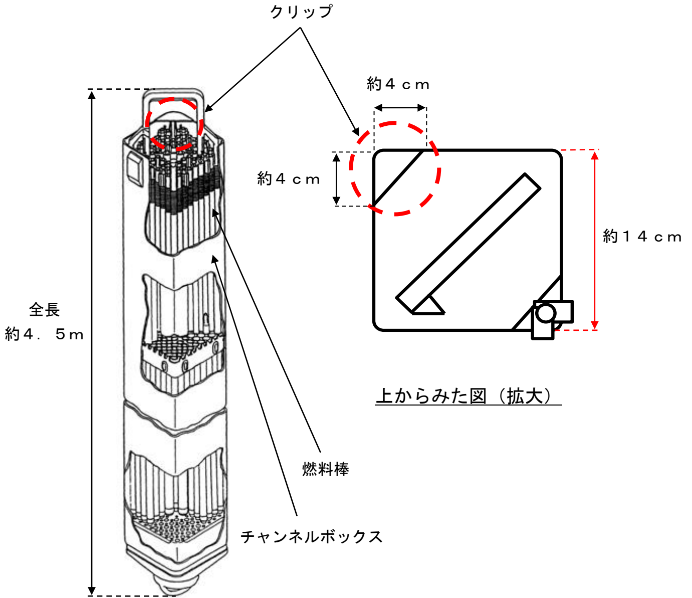
燃料集合体概要図
