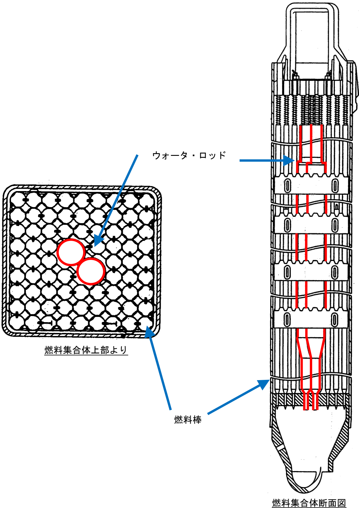
燃料集合体ウオータ・ロッド概略図 (9×9燃料の例)
